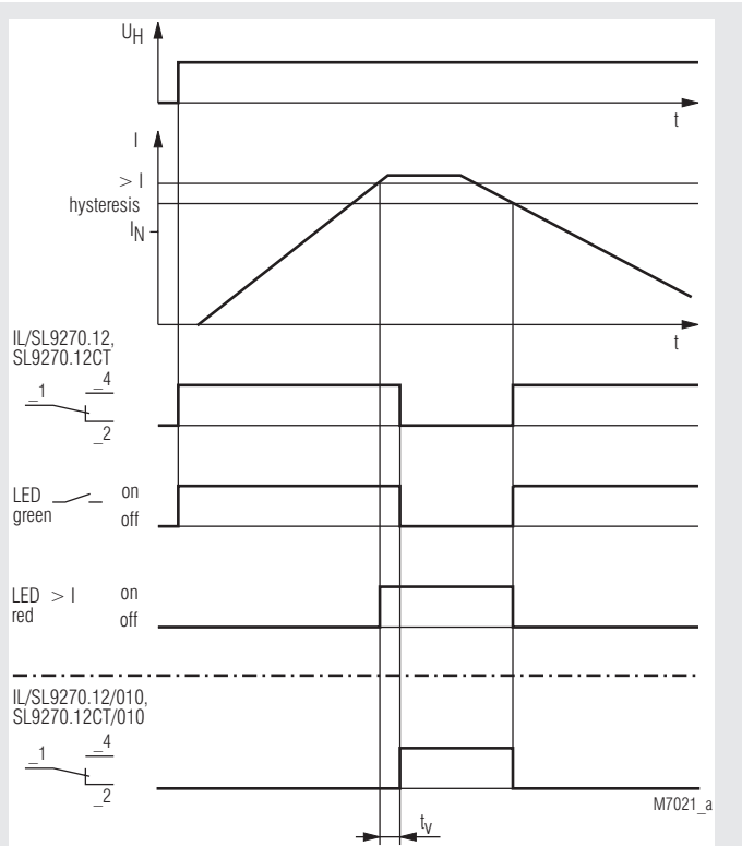
Function Diagram IL 9270.12, SL 9270.12
